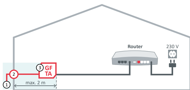
Abbildung 1: Beschreibung Glasfaser-Hausanschluss
